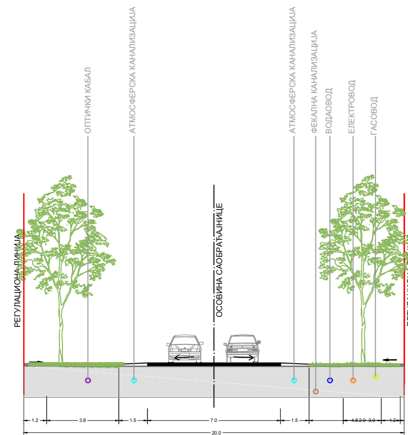
ПРЕСЕК 5-5 ул. НОВА 5
