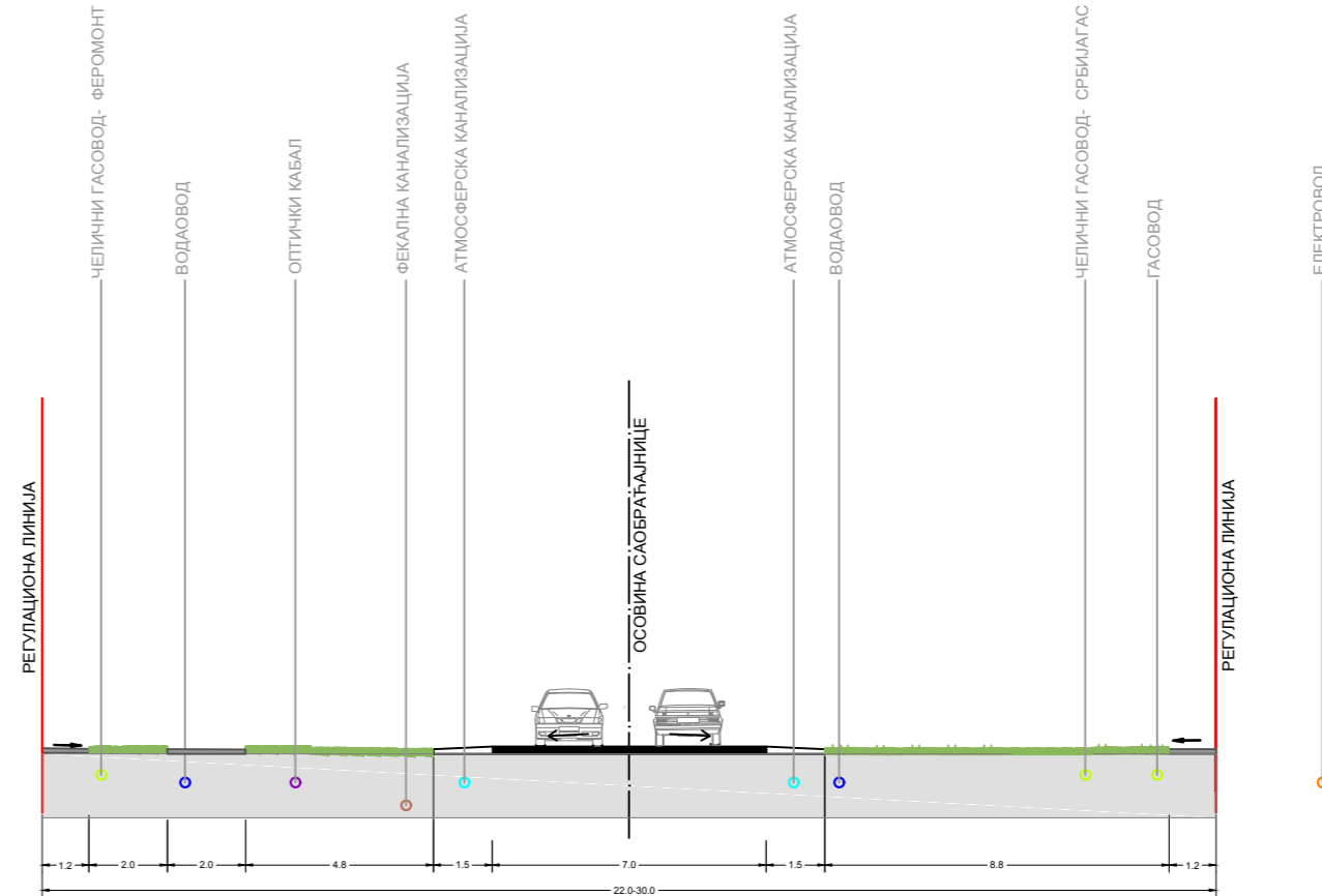
ПРЕСЕК 4-4 ул. ИНФРАСТРУКТУРНИ КОРИДОР
