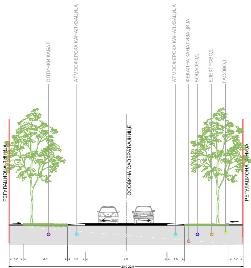
ПРЕСЕК 7-7 ул. НОВА 8,14,15,16,17,18,19 И 21
