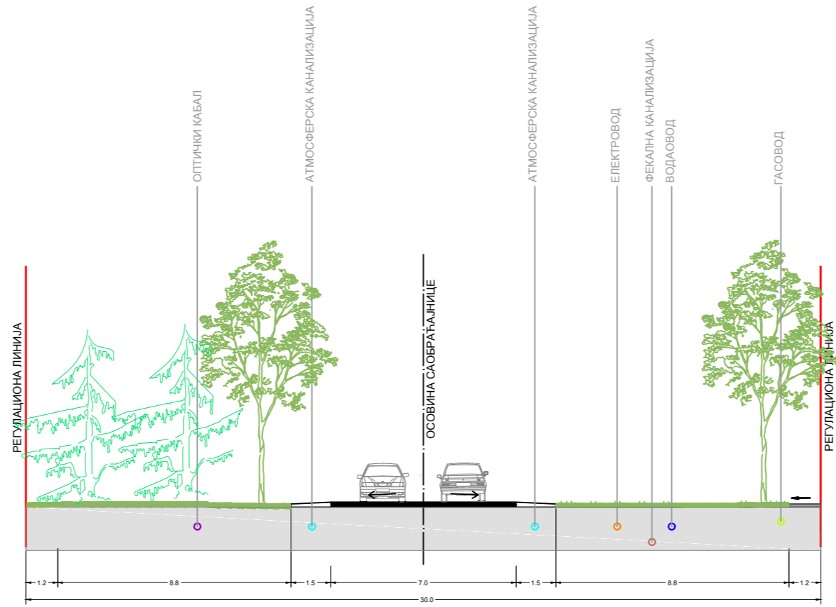
ПРЕСЕК 3-3 ул. ИНФРАСТРУКТУРНИ КОРИДОР
