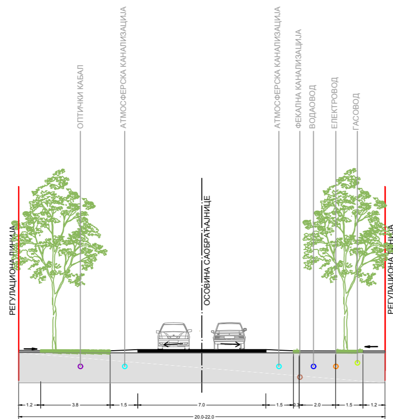
ПРЕСЕК 6-6 ул. НОВА 7,8,12 И 13
