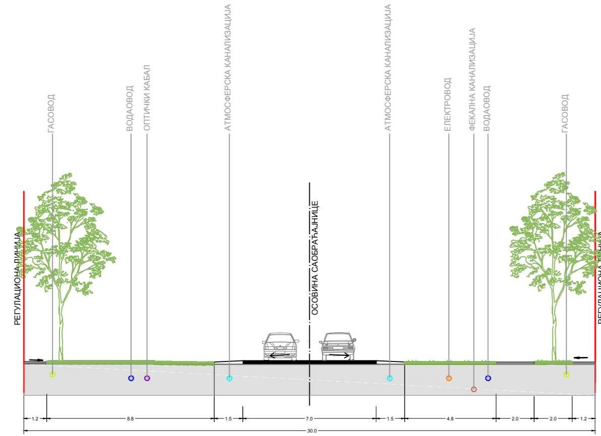
ПРЕСЕК 1-1 ул. ПРВА И ДРУГА ЦЕНТРАЛНА ЗПНА, ЈУЖНА РАДНА, НОВА 1,2,3,4,9,10 И 11
