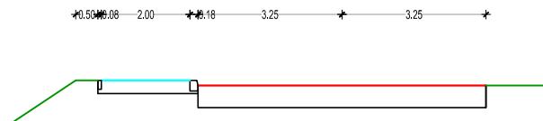
ПРЕСЕК 16-16
