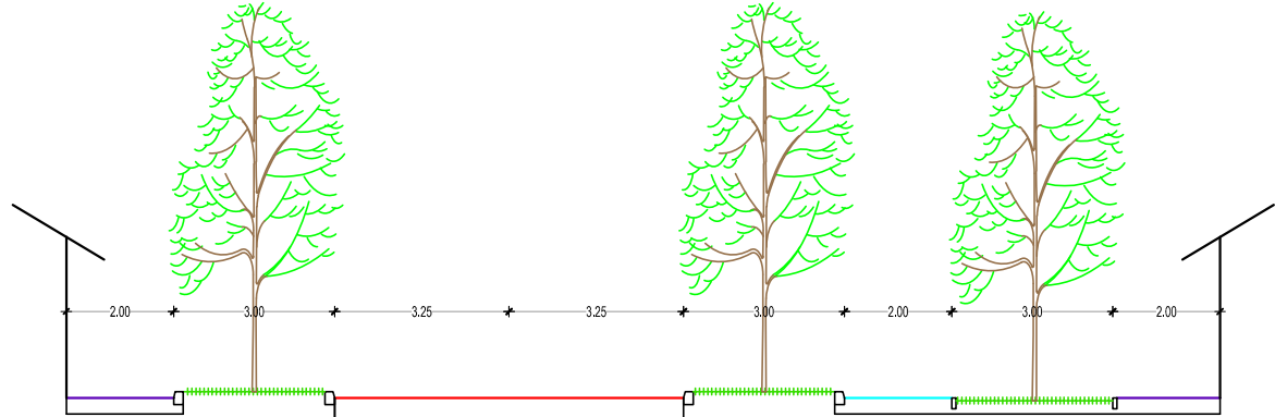
ПРЕСЕК 5-5 Петроварадин (Прерадовићева од Роковог потока до Карловачког друма - окретница аутобуса)
