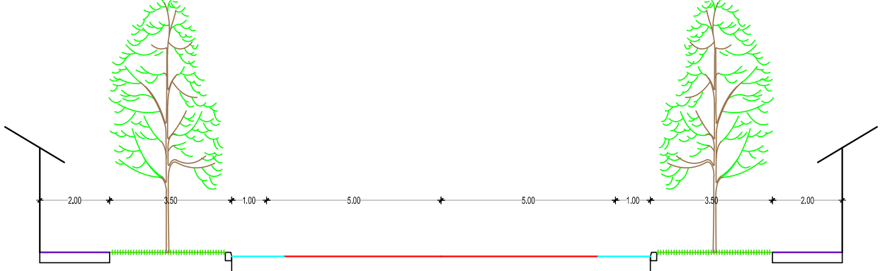
ПРЕСЕК 3-3 Петроварадин (Прерадовићева улица до пијаци)
